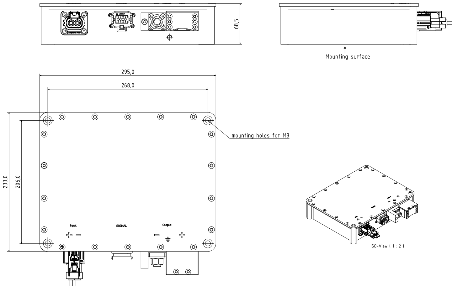
Abbildung 8.1: Abmessungen
