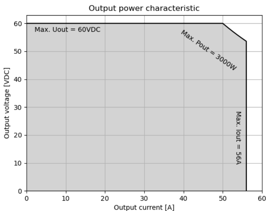
Abbildung 9.3: Ausgangsleistung DVCH3003-700-48
