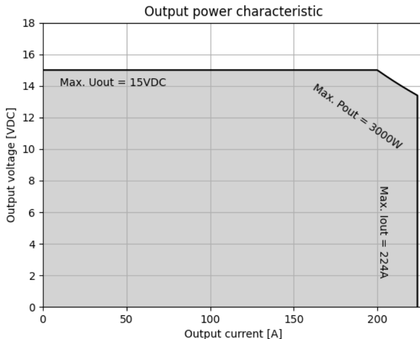
Abbildung 9.1: Ausgangsleistung DVCH3003-700-12
