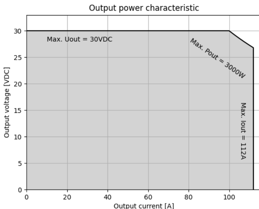
Abbildung 9.2: Ausgangsleistung DVCH3003-700-24
