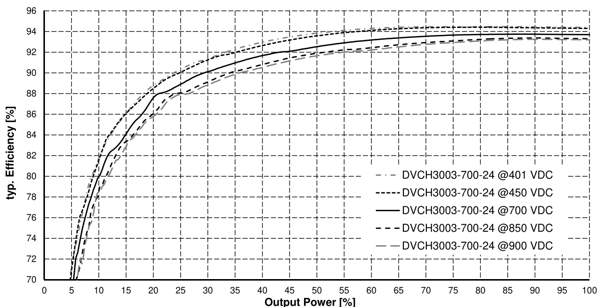
Abbildung 9.4: Wirkungsgrad in Abhängigkeit der Ausgangsleistung
