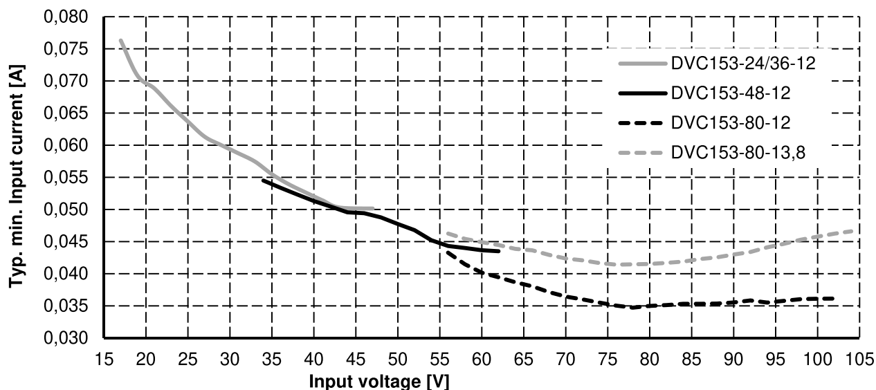
Abbildung 9.2: Leerlaufstromaufnahme in Abhängigkeit der Eingangsspannung
