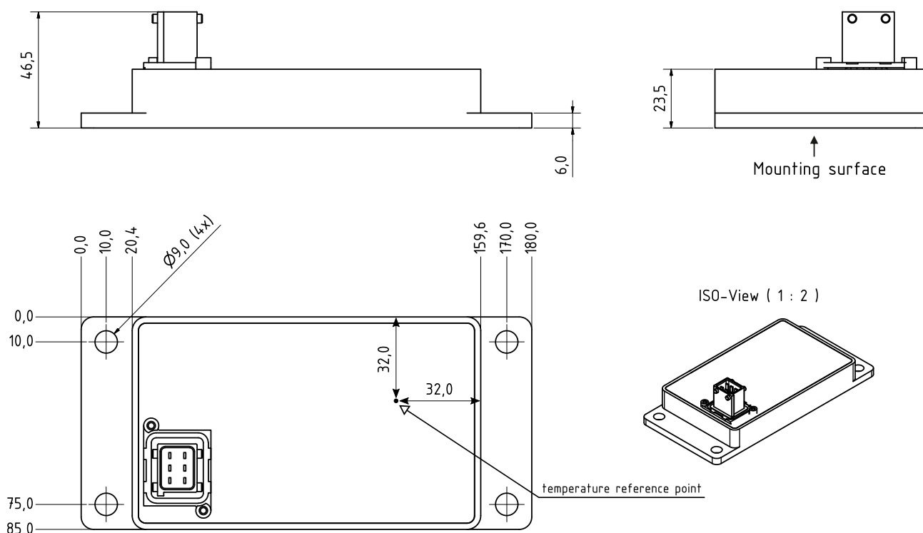
Abbildung 8.1: Abmessungen
