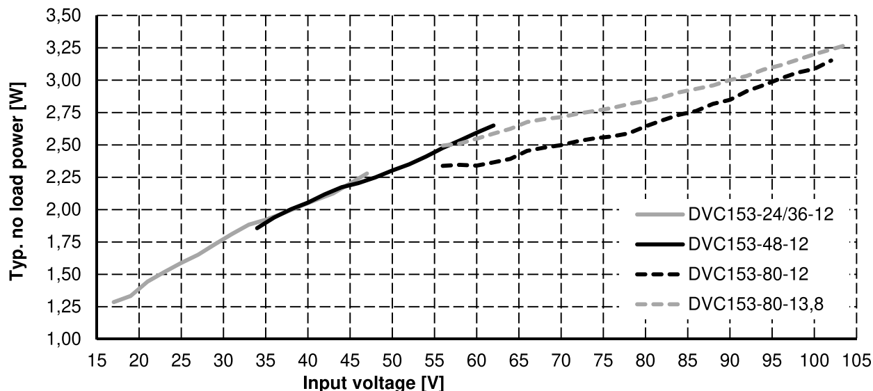
Abbildung 9.1: Leerlaufleistung in Abhängigkeit der Eingangsspannung
