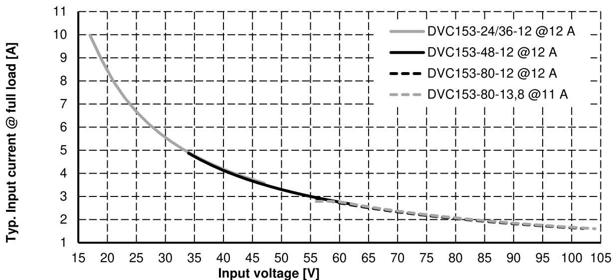
Abbildung 9.3: Stromaufnahme bei Vollast in Abhängigkeit der Eingangsspannung
