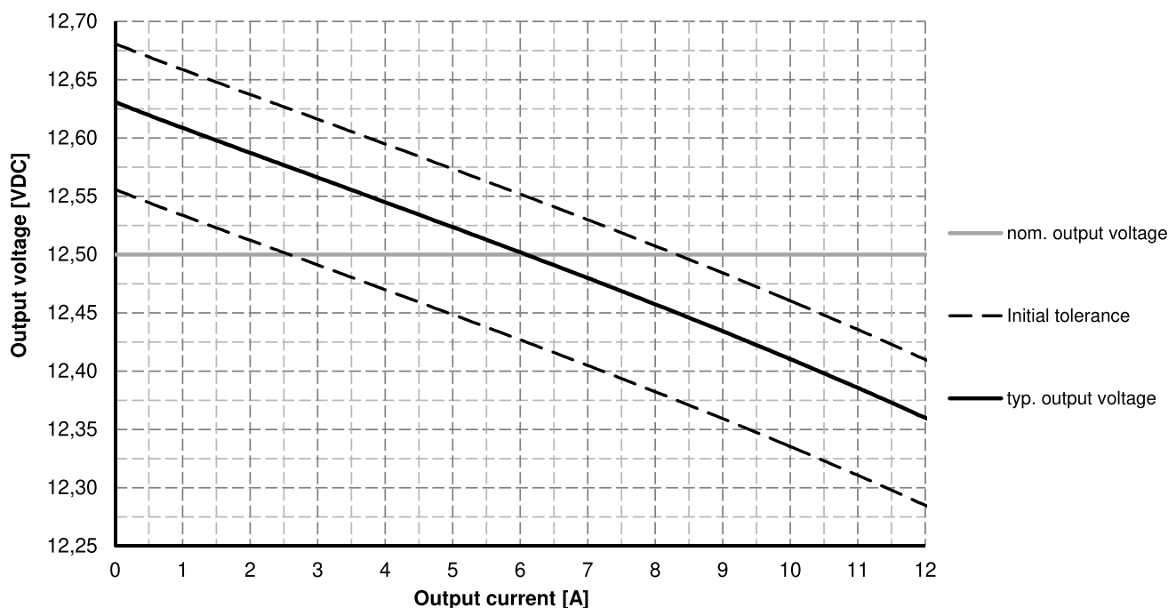
Abbildung 9.8: Typ. Ausgangsspannung und Initialtoleranz ( U_{nom}=12,5 VDC)
