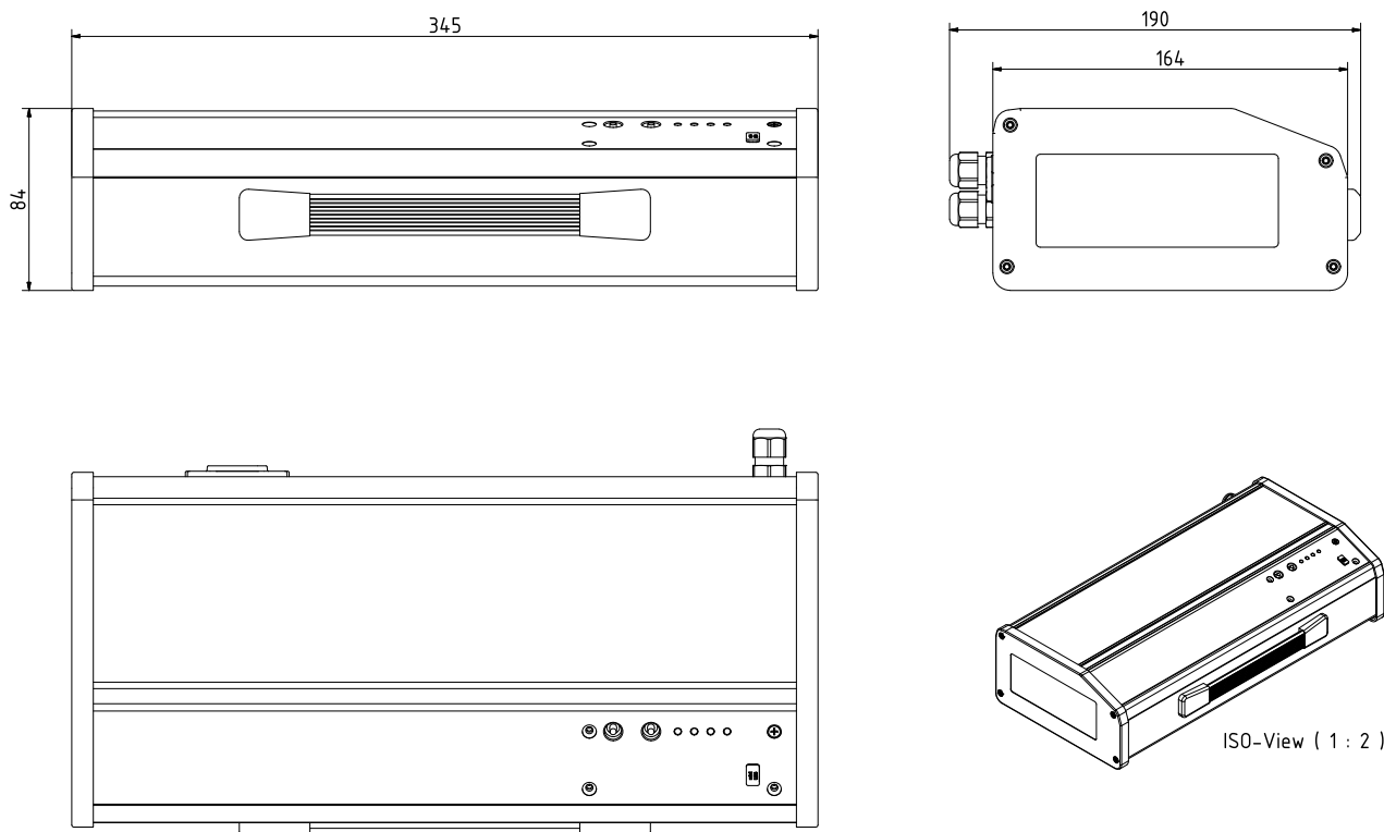
Abbildung 7.1: Abmessungen
