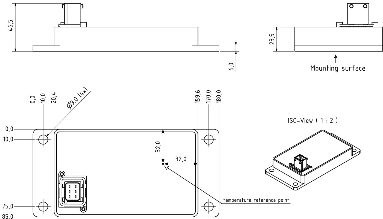
Abbildung 8.1: Abmessungen
