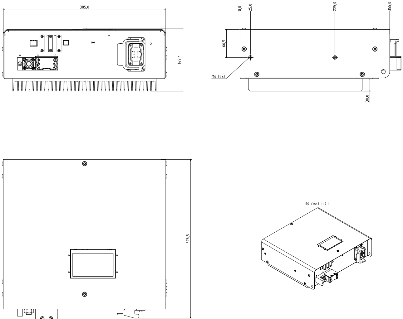
Abbildung 8.1: Abmessungen
