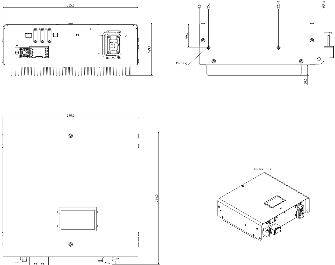
Abbildung 8.1: Abmessungen
