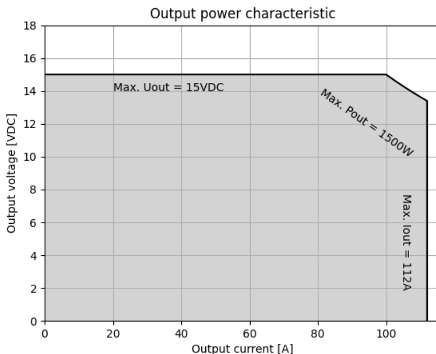
Abbildung 9.2: Ausgangsleistung DVCH1503-400-12
