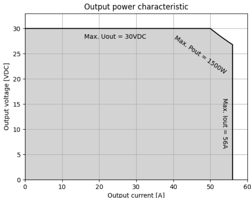
Abbildung 9.1: Ausgangsleistung DVCH1503-400-24
