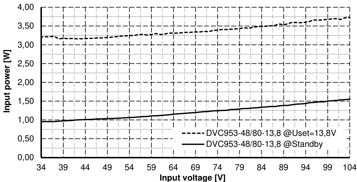
Abbildung 10.2: Leerlaufleistung
