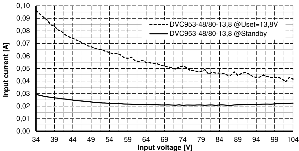
Abbildung 10.1: Leerlaufstromaufnahme
