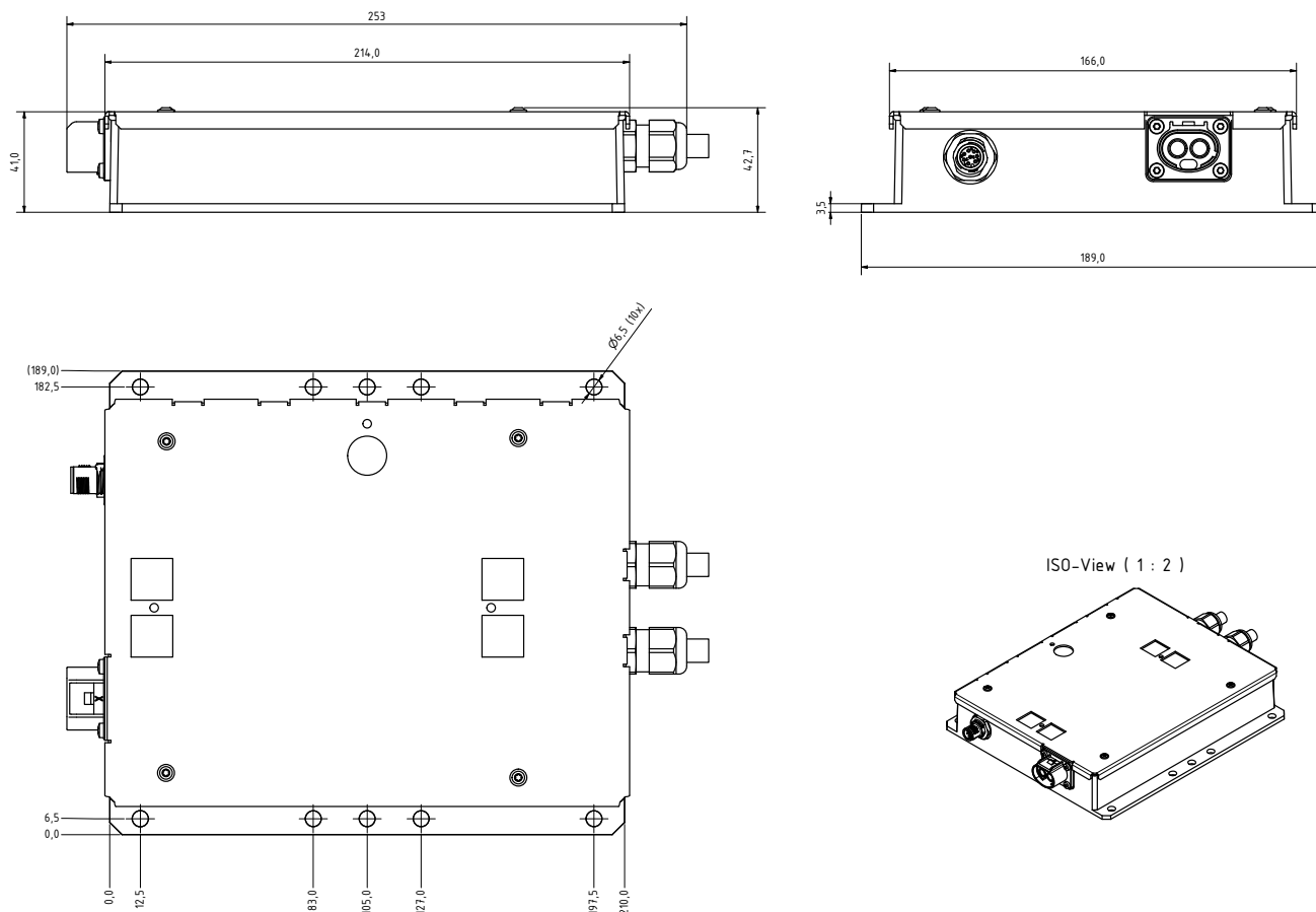
Abbildung 9.1: Abmessungen
