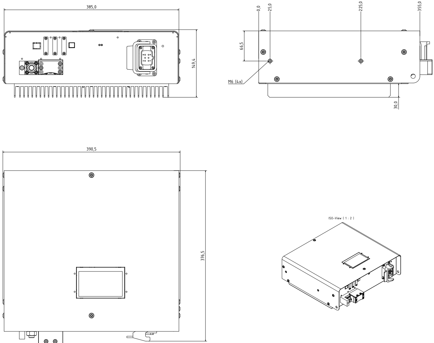
Abbildung 8.1: Abmessungen
