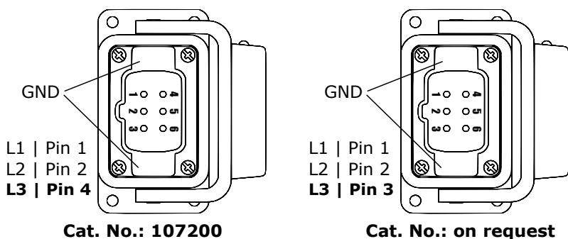
Abbildung 8.2: Pin-Belegung Anschluss Eingang
